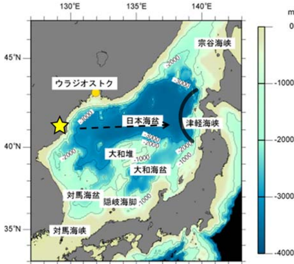
Fig. 3 Bathymetry of the Japan Sea (日本海海洋気象センターの図に加筆)
