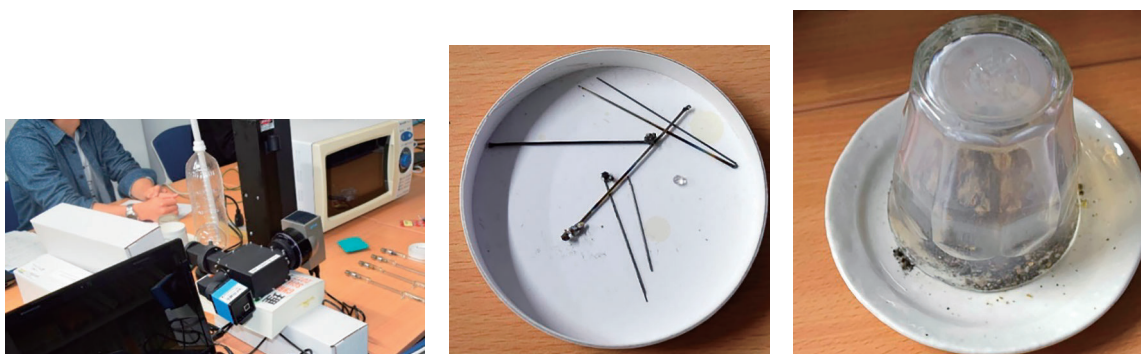
図1. (左) 実験に用いた電子レンジが右上, 中央に分光器がある. (中央) アンテナとして用いたシャープペンの芯と待ち針. シャープペンの芯は両端がやせ細り, 待ち針の両端は高温で溶けて固まりができています. (右) アンテナとして用いるシャープペンの芯や待ち針を高温に耐えられる陶器の皿にのせ, 耐熱コップをかぶせて, プラズマ閉じ込めの容器とする.
