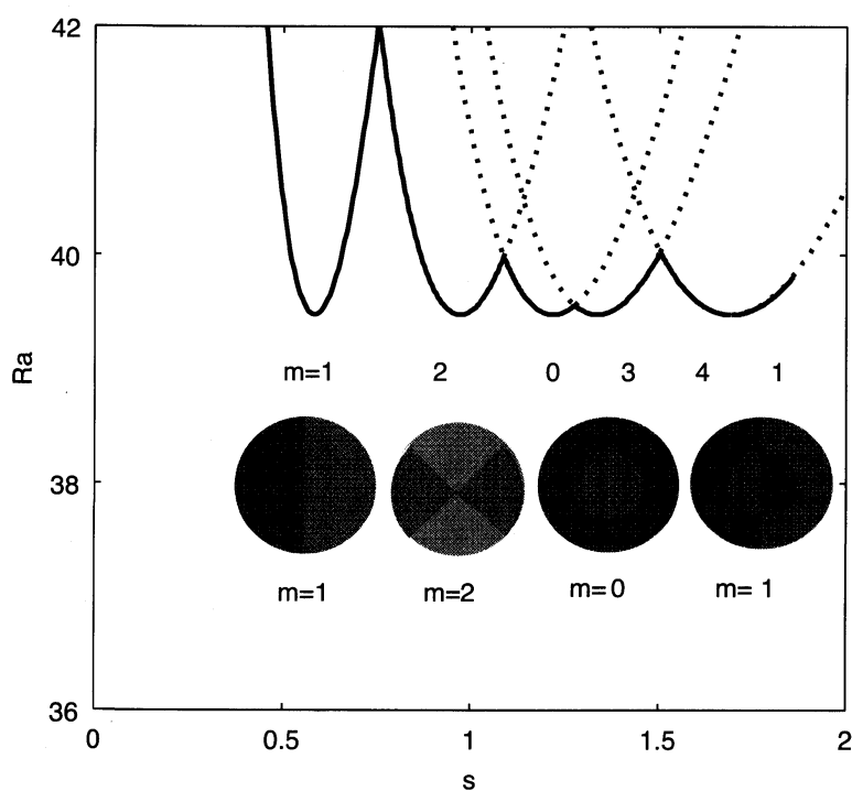
図 2: Rayleigh 数 ( Ra ) とアスペクト比 ( s ) における中立安定曲線と対流モード：図中各モード m における対流パターンの色違いは上昇流と下降流に対応する。
