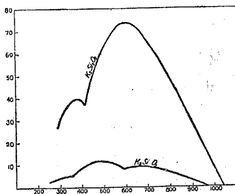
H_2O と K_2SiO_3 との作る溶液における 溫度(横軸) 壓力(縦軸氣壓)平衡曲線
