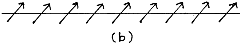
図 31 スピン秩序状態 (a) J_z > J_{\perp} , (b) J_z < J_{\perp}
