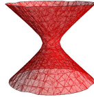
図2 ド・ジッター空間
