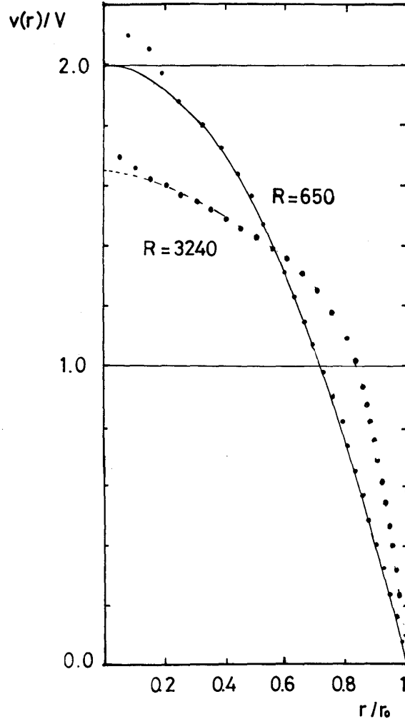
第7図 Hagen Poiseuille 流の速度の空間分布と R = 3240 の乱流の速度の空間分布。実線は(18)を表わす。破線は r=0 で dv/dr = 0 を考慮してひいた。
