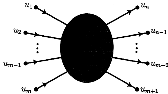
図 1: n 点 Green 関数 \mathcal{G} に対応する Feynman 図形
