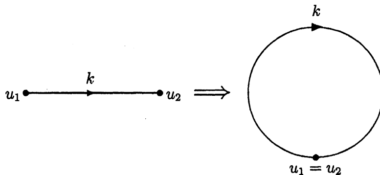
図 11: k 次の伝播関数 g^{(k)} から作られるループ図形
