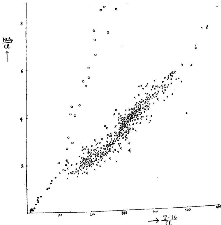
第 3 圖 別府市内温泉の \frac{\text{HCO}_3}{\text{Cl}} と \frac{T-16}{\text{Cl}} の關係 ● 第一地域 ○ 第二地域 × 第三地域
