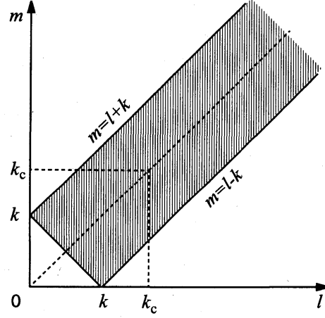
図1 陰影をつけた領域は、波数 k, l, m が三角形 k + l + m = 0 を形成できるような (l, m) 平面の領域。三波エントロピー伝達関数 T_\alpha^Q(k, l, m) は陰影をつけた領域以外ではゼロである。
