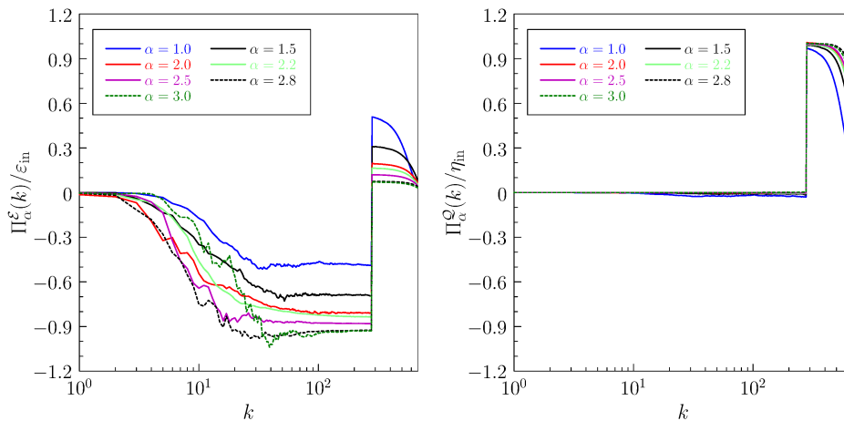
図 3 左図：直接数値実験から得られたエネルギーフラックス。エネルギー注入率 \varepsilon_{\text{in}} で規格化している。凡例は図に示してある。右図：直接数値実験から得られたエントロフィーフラックス。エントロフィー注入率 \eta_{\text{in}} で規格化している。凡例は図に示してある。
