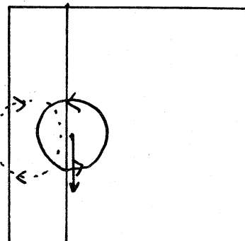
(a) 惑星ベータ効果 (b) 地形性ベータ効果 (c) 鏡像効果
