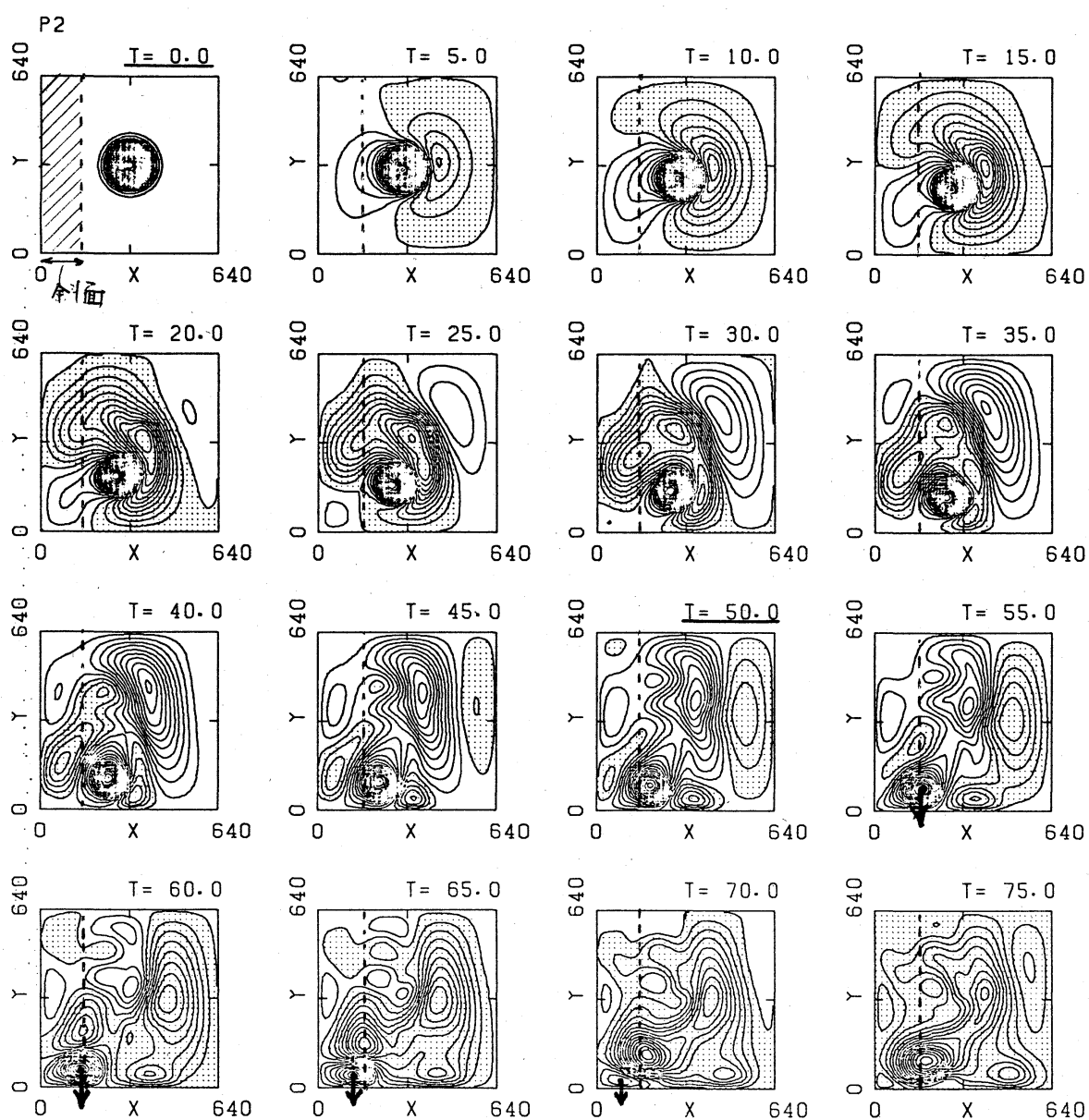
図3(b) Case Bの下層の圧力分布.
