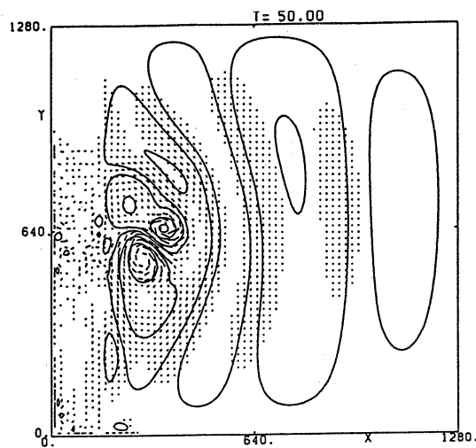
(b) 高気圧性渦
