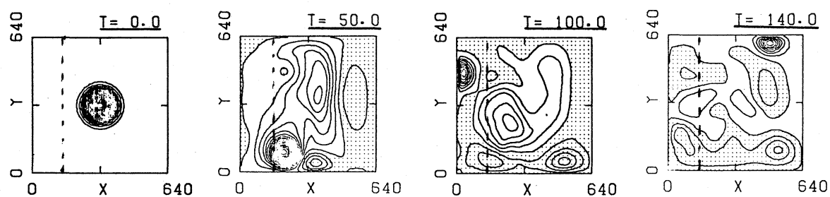
図3(a) Case Bの上層の圧力分布.
