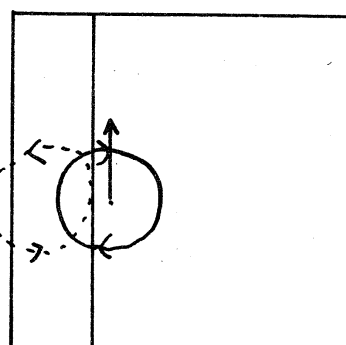
図1. 渦の移動に関する模式図. 矢線は渦の移動方向を示す.
