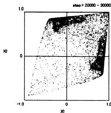
図 9-1: H_{55} 上の軌道
