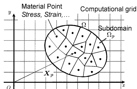
図-1 Material Point Method の概念図
