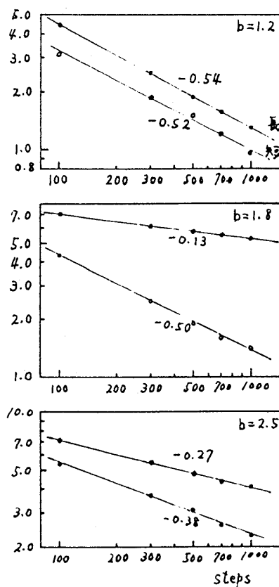
図3 Modified Bernoulli一次元写像の規格化ピアソンイメージの収束速度。パラメータ値は b = 1.2, 1.8, 2.5 。黒丸は左右方向の長さ、白丸は上下方向の長さの収束を調べたものである。イメージは左右方向に細長くなっている。横軸はステップ数、たて軸はイメージの各方向の長さを表す。たて軸の単位は適当に選んである。
