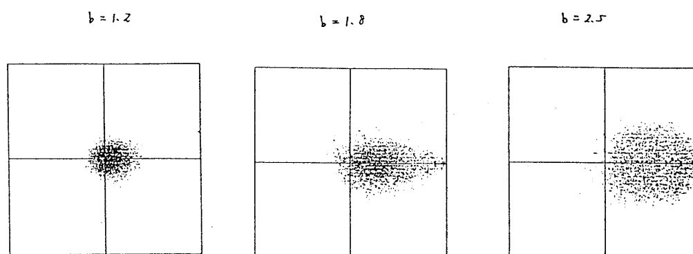
図 1 100 step のときの Modified Bernoulli 一次元写像の規格化ピアソンイメージ。パラメータ値は b = 1.2, 1.8, 2.5 である。
