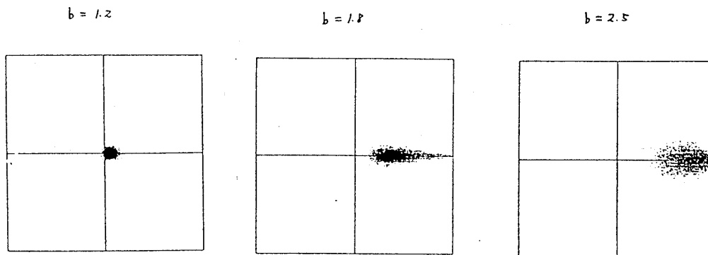
図2 1000 stepのときのModified Bernoulli一次元写像の規格化ピアソンイメージ。パラメータ値は b = 1.2, 1.8, 2.5 である。
