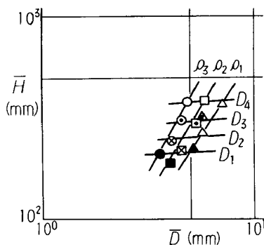
図8 要因方向の相対生長関係の例 スギ苗を利用した生育実験の結果をしめしてある。土壌の深さ D_i ごとに, 植栽密度 \rho_j ごとに別の相対生長関係がはっきりでている。(青山 3) による。)
