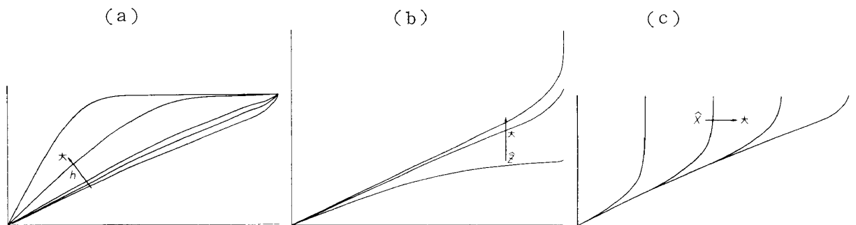
図7 \frac{1}{z} = \frac{1}{C\hat{Z}} \left( \frac{\hat{X}-x}{x} \right)^h + \frac{1}{\hat{Z}} の両対数軸にあらわす曲線群
