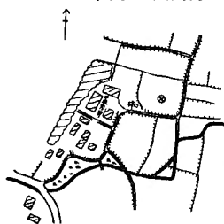
No. 69 上木場其の6 門小屋西南方
