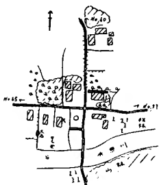
No. 61 中木場 其の5
