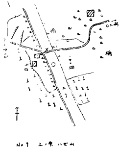
No. 9 上の原ハゼ山土手上
