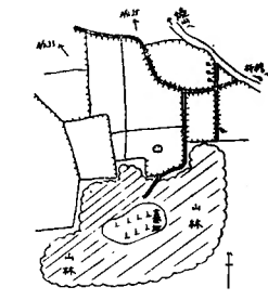
No. 34 北千本木町其の4 墓地北方
