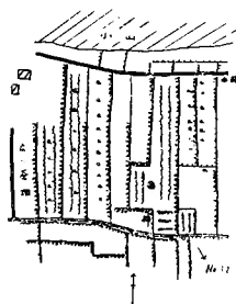
No. 31 北千本木町其の1 茶畑の間
