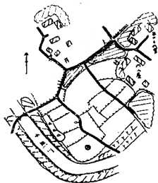
No. 69 上木場其の6 門小屋西南方
