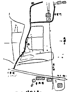
No. 10 護国寺西方小丘上
