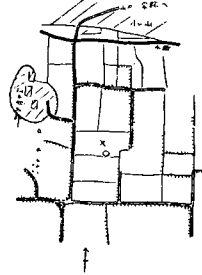
No. 37 北千本木町其の7 松本初太郎方東南
