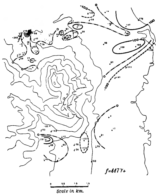
第15図 全磁力の長期変化 (1923. 50~1952. 63)
