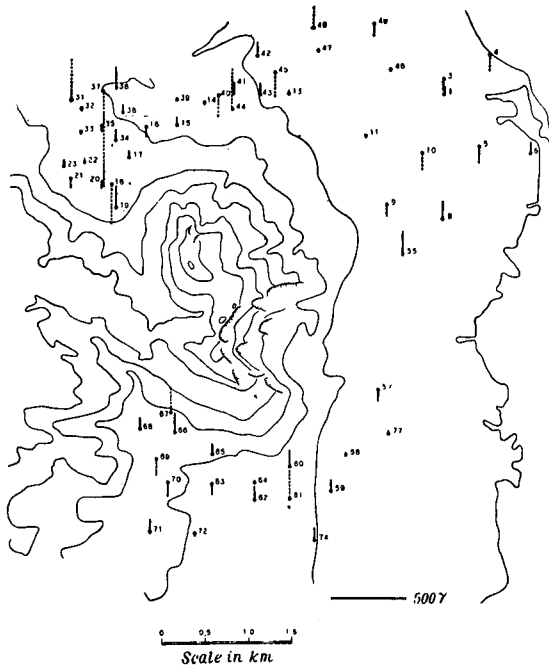
第20図 局地異常の垂直分力の増加, 但点線は式を出す時除外した点のもの。
