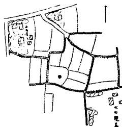
No. 68 上木場其の5 園田利八郎西南方
