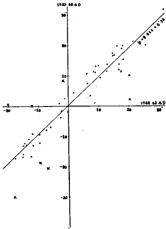
第19図 1923. 50の \Delta V と1952. 63の \Delta V との関係
