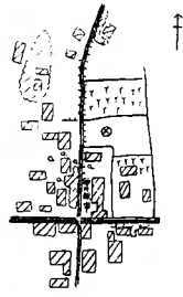
No. 58 中木場 其の2 元小学校々庭跡
