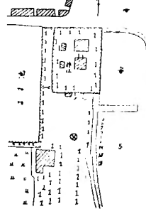
No. 4 猛島神社境内
