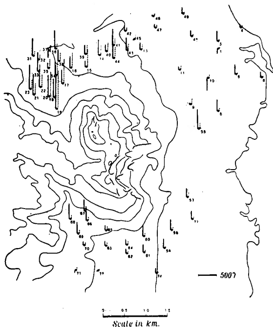
第9図 第二次異常 (1952.63, 上下方向) (実線は測定値, 破線は計算値)
