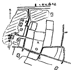
No. 67 上木場其の4 岩崎カヒ北西方
