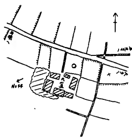
No. 43 下折橋其の1 丸山直北方
