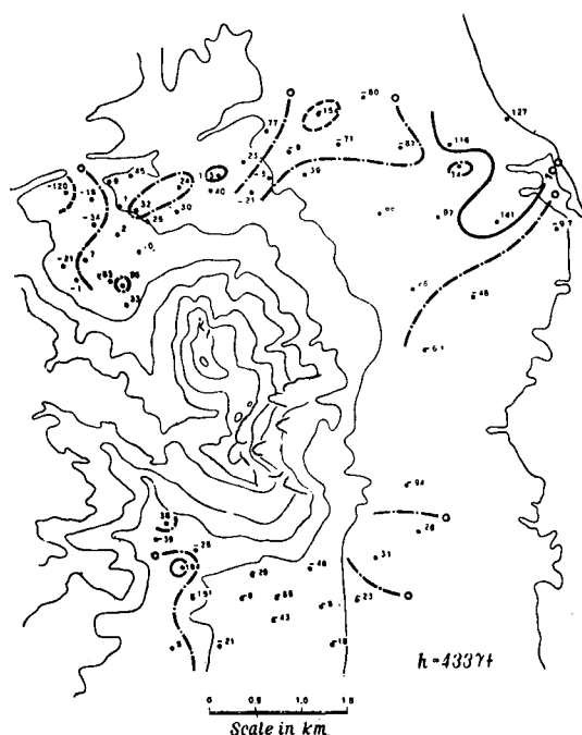
第13図 水平磁力の長期変化 (1925. 30—1952. 63)
