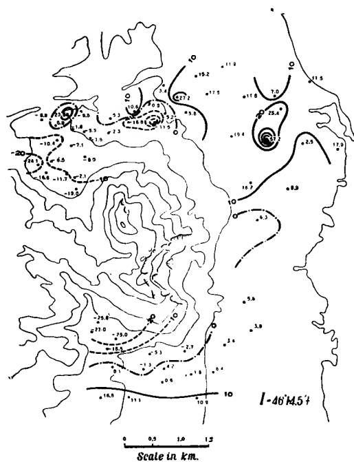
第6図 1952.63に於ける全磁力の分布
