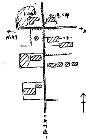
No. 46 上新町吉田 近恭南方
