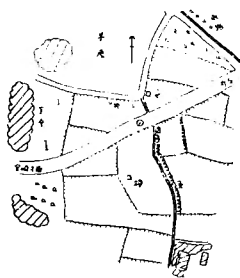
No. 20 千本木町其の4 道路上
