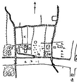
No. 59 中木場 其の3 佐藤豊次東北
