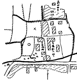
No. 60 中木場 其の4 寺田福松西方
