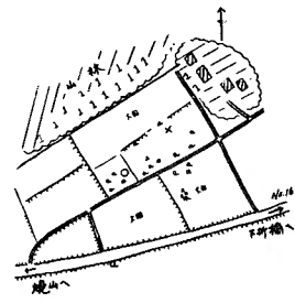
No. 38 北千本木町其の8
