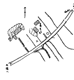
No. 41 六木其の1 宮崎厚方
