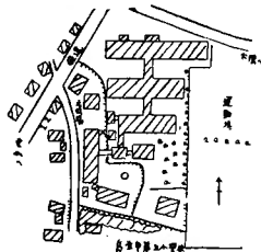
No. 77 中木場其の7 島原市立第九小学校
