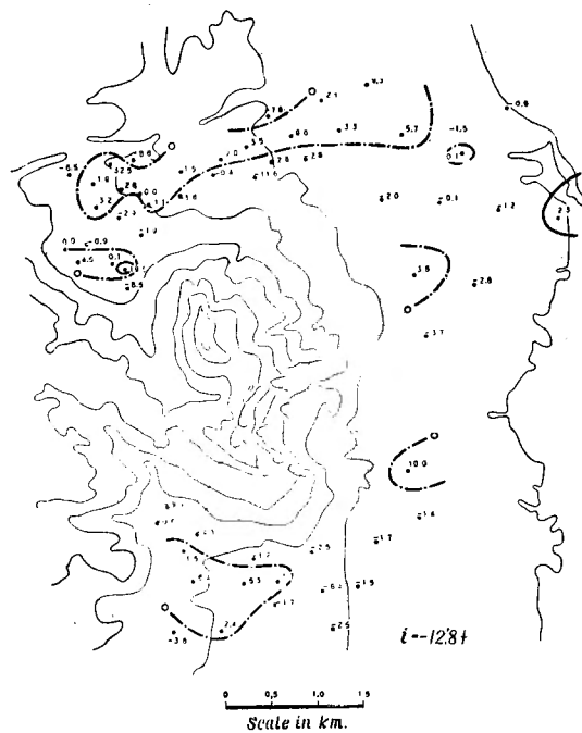
第15図 全磁力の長期変化 (1923. 50~1952. 63)
