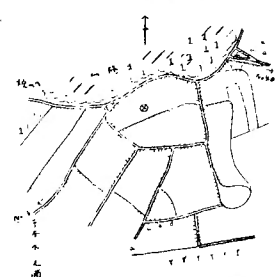
No. 39 上折橋荒木方 西北方
