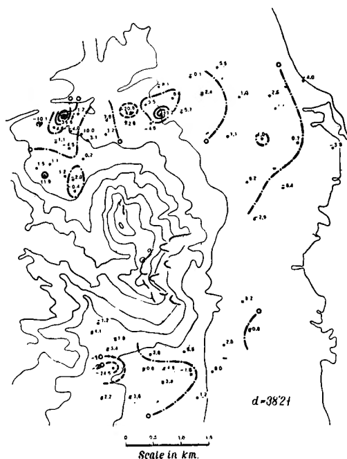
第12図 偏角の長期変化 (1923.50—1952.63)
