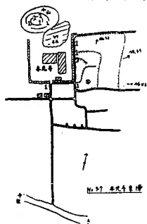
No. 47 本光寺東方
