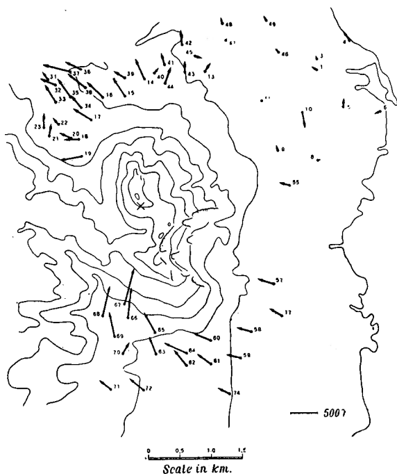
第 7 図 第一次異常 (1952. 63 水平方向) (数字は測点番号)
