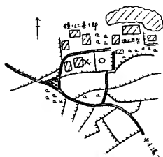
No. 65 上木場其の2 坂上年男西方
