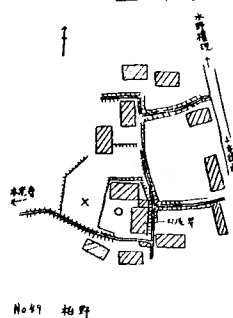
No. 49 柏野村尾昇西方
