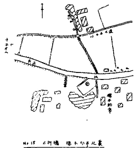
No. 15 上折橋、橋本助市 北裏
