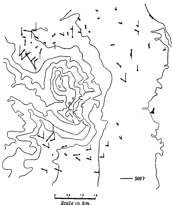
第11図 第三次異常
