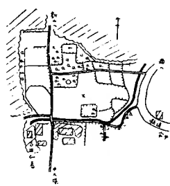
No. 57 中木場 其の1
