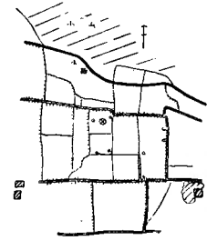
No. 36 北千本木町其の6
