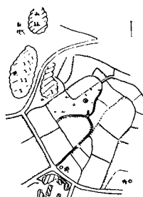
No. 22 千本木町其の6 堀川浅造方北東方
