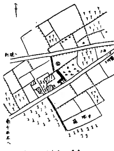
No. 16 千本木入口 元酒店北
