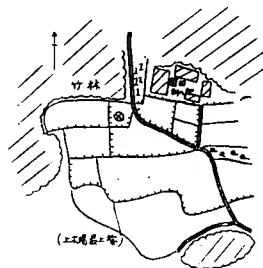
No. 68 上木場其の5 園田利八郎西南方
