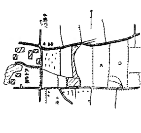
No. 62 大野木場其の1 大山蔵東方
