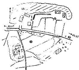
No. 66 上木場其の3 谷口富士吉東方
