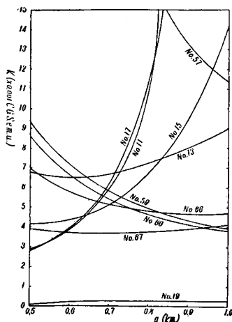
第10図 楕円体の短軸( a )と磁化率( K )との関係 ( \Delta H の場合)但し測点10個に就いて
