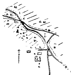
No. 67 上木場其の4 岩崎カヒ北西方
