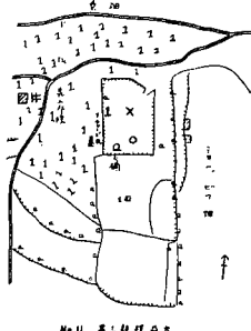
No. 11 甚三郎様(社) 東方
