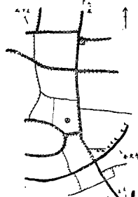
No. 45 六木其の3 墓の北方
