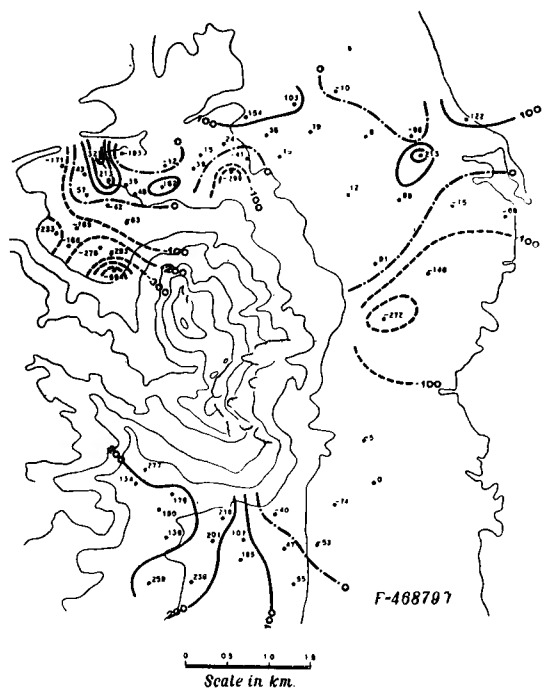
第6図 1952.63に於ける全磁力の分布
