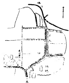
No. 35 北千本木町其の5 片山忠次郎東方
