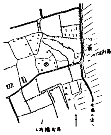
No. 40 上折橋部落 北方丘上
