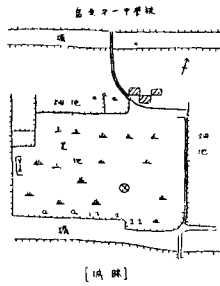
No. 3 旧島原村高等 小学校跡
