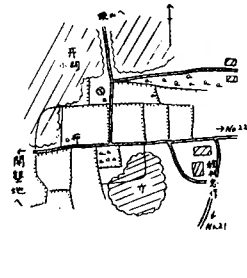
No. 23 千本木町其の7 種村忠作方北西方
