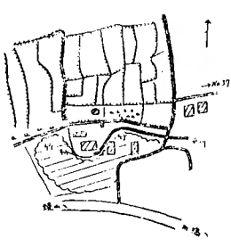
No. 32 北千本木町其の2
