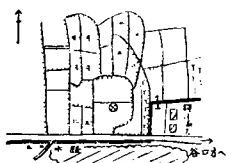
No. 70 上木場其の7 鐘ヶ江満吉西方
