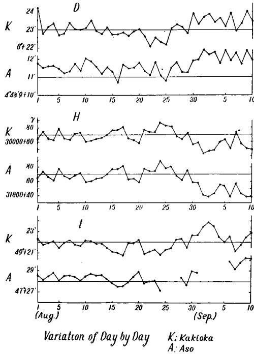
第1図 阿蘇及び柿岡に於ての逐日変化
