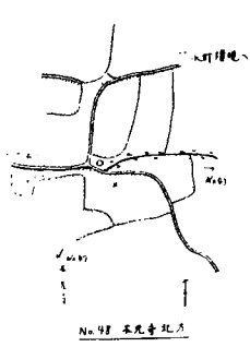
No. 48 本光寺北方
