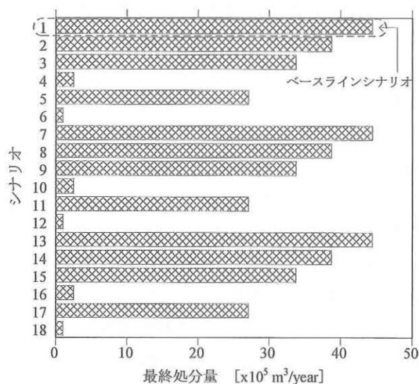
図-7 各シナリオにおける最終処分量
