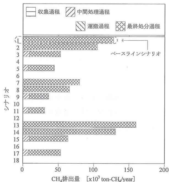
図-5 各シナリオにおける \text{CH}_4 排出量
