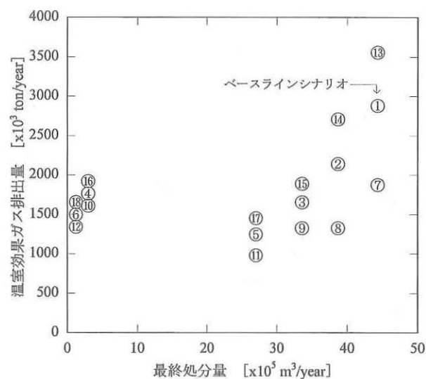
図-8 各シナリオにおける最終処分量と温室効果ガス排出量の関係
