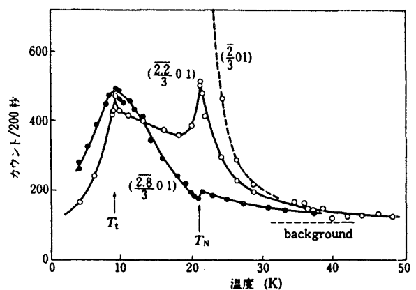
図3 \text{CsCoCl}_3 の中性子臨界散乱
