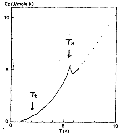
図9 RbFeBr 3 の比熱
