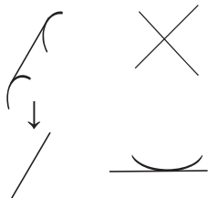
FIGURE 1. 折り目写像の特異点集合の一部と像 (左), 特異値集合の一部分と像 (平面への場合で右上が安定な場合右下が不安定な場合).
