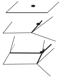
FIGURE 8. pseudo spherical 写像で値域が 2 次元の場合の局所的な形 (太い線が特異値集合の一部分を表す)
