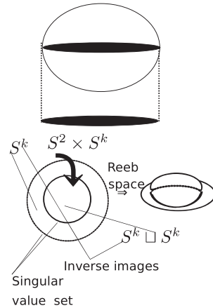
FIGURE 7. 具体的な折り目写像と Reeb 空間
