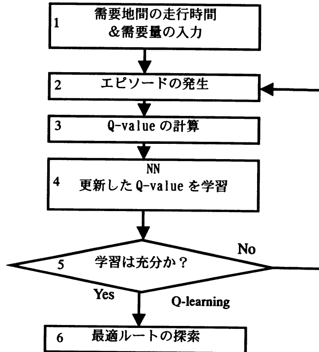
図3 本技法のフローチャート
