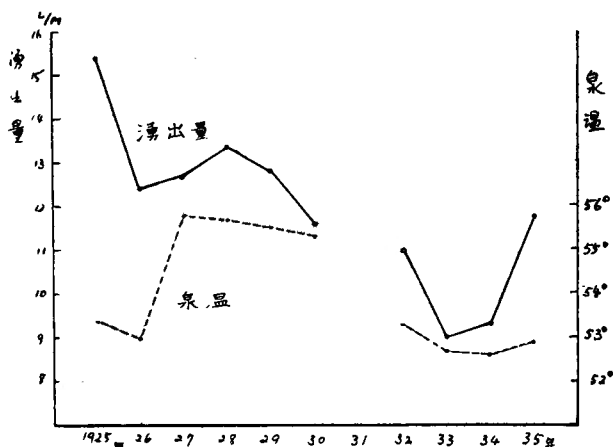
第4圖 別府温泉8口平均の永年変化
