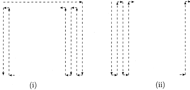
図 3 : comprehensive path
