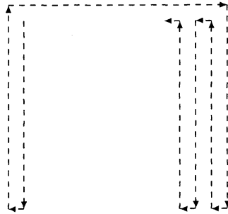
図 4 Hamilton 閉路
