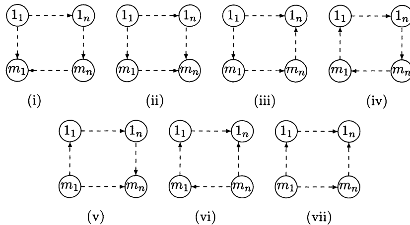
図2 周の可能性
