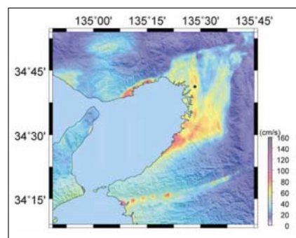
図1、南海地震(M8.4)時に予測される地震動強さの分布
