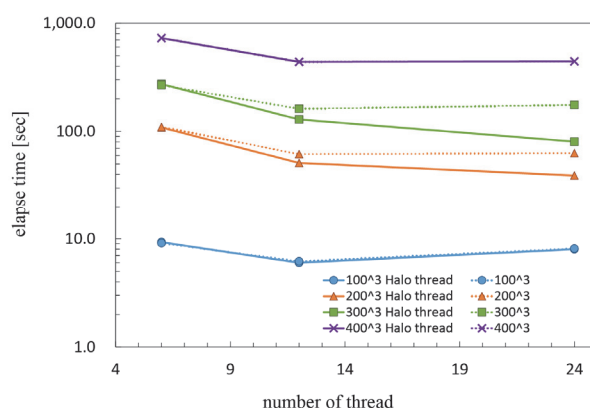
図 6 HA8000 における計算サイズとスレッド数変化時の Halo スレッドの効果
