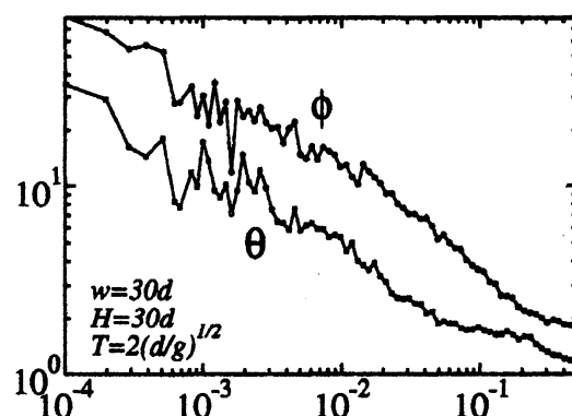
Figure 6: 3次元の砂山について、頂点の方向 \phi と \theta のパワースペクトル。 w = 30d, H = 30d, T = 2\sqrt{d/g} 。線が重なるため \theta についてのプロットを下にずらした。
