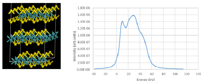
図2 MoS 2 の結晶モデルおよび第一原理計算による XAFS プロファイル
