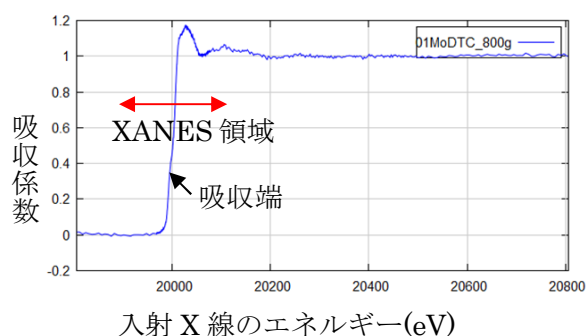
図1 Mo-K 吸収端近傍 XAFS プロファイル
