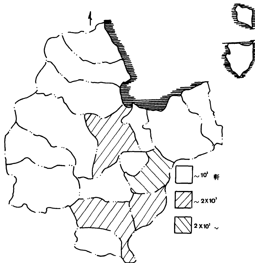
図6-2 1988年11月災害における家屋被害分布図
