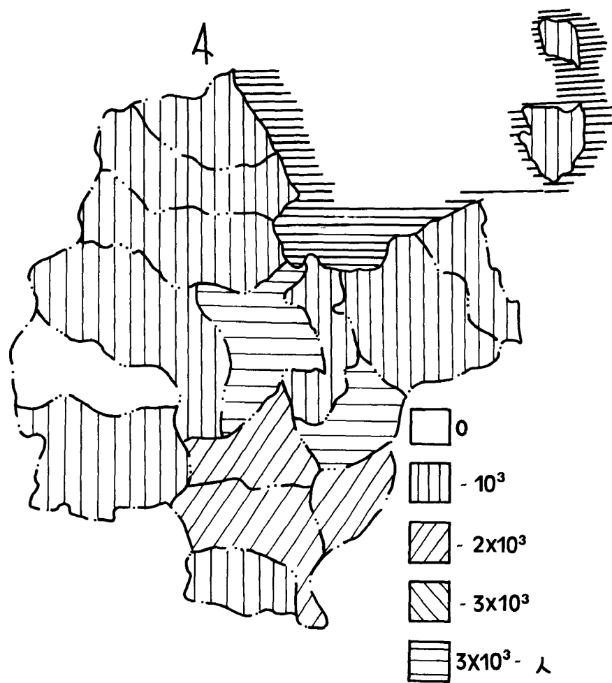
図6-1 1988年11月災害における被災者分布図
