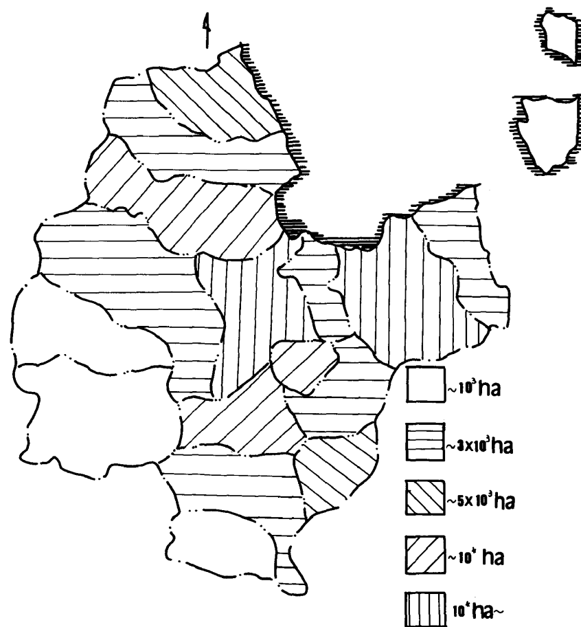
図 6-4 1988年11月災害における農地被害分布図
