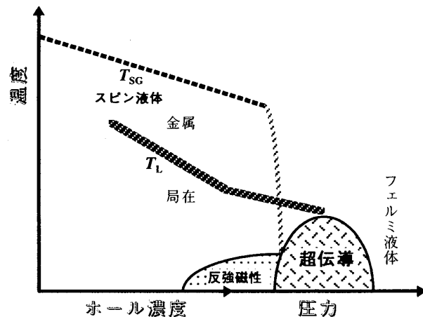
図 12: \text{Sr}_{14-x}\text{Ca}_x\text{Cu}_{24}\text{O}_{41} における二本足梯子格子の相図の概念図。 T_{SG} はスピニングギャップ形成温度、 T_L はキャリアが局在する温度 ( d\rho_c/dT=0 ) を表す。
