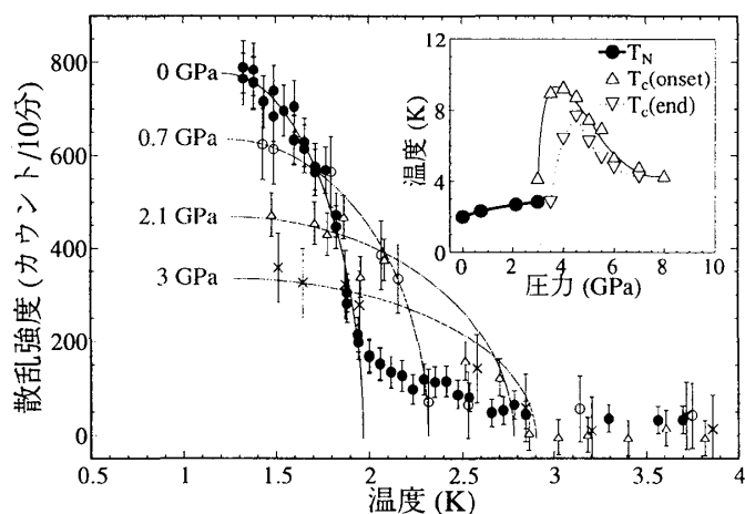
図 11: \text{Sr}_{2.5}\text{Ca}_{11.5}\text{Cu}_{24}\text{O}_{41} の磁気ブラッグピーク (1 0 12) の様々な圧力におけるピーク強度の温度依存性。挿入図は反強磁性転移温度と電気抵抗率から見積もられた超伝導転移温度の圧力依存性。
