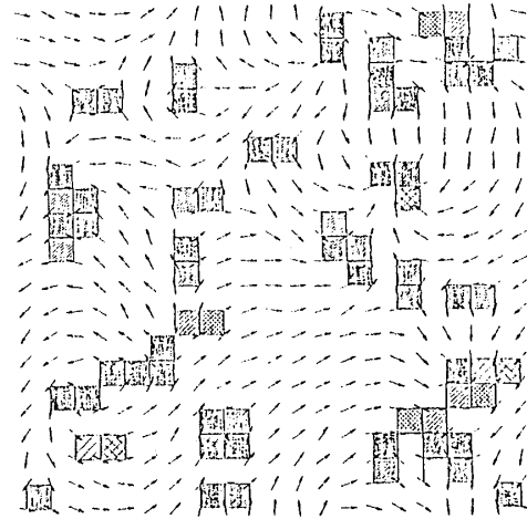
図2 カイラリティ及びスピンのスナップショット。温度 T=0.1 J。ランダムな初期スピン配位から 10^4 MCS 後のショット。太線が反強磁性ボンド、ハッチ(クロスハッチ)された正方形は+(−)のカイラリティを持つ。白いプラケットはカイラリティがほぼ0のもの( |\kappa| < 0.2 )を表わす。系のサイズは 20 \times 20 。さらに大きな系( 40 \times 40 , 100 \times 100 )でも類似のサイズの渦が観測された。
