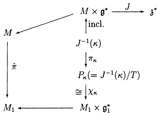
図 1: 力学系の簡約
