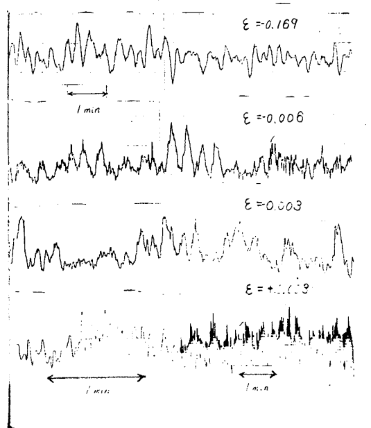
図 4-1 フォトマルの出力電流 (臨界点に近づくにつれ振動が早くなるのでわかる。)
