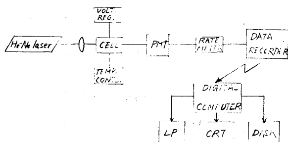
図 3 光学系・処理系
