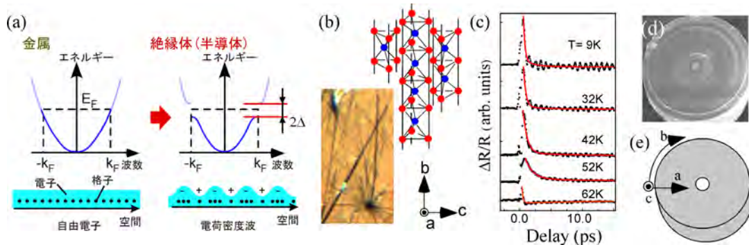
図 12: (a) パイエルス転移の概要。(b) 擬一次元結晶 \text{NbSe}_3 の結晶構造。一般的には写真に示すような針状結晶となる。(c) 針状結晶で得られる過渡反射率変化 \Delta R の温度依存性。低温で見られるコヒーレント振動は電荷密度波 (CDW) の集団励起。(d) ディスク型 \text{NbSe}_3 リング結晶と (e) その結晶軸。
