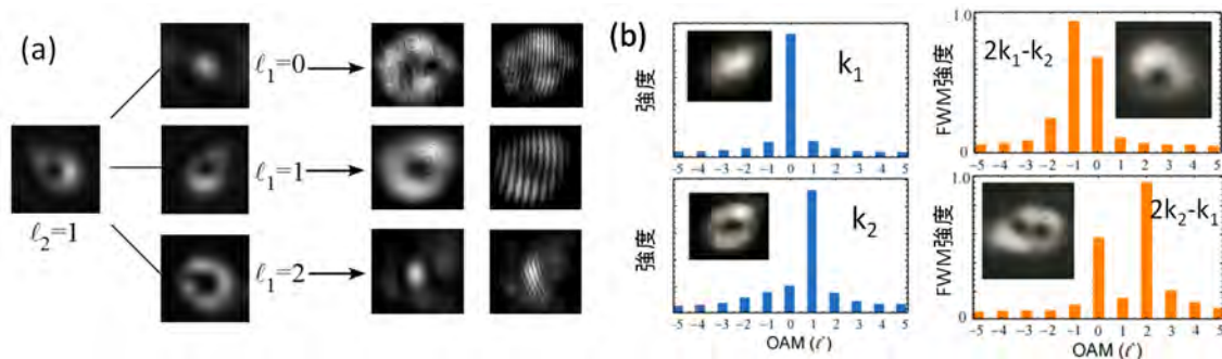
図 10: (a) 異なるトポロジカルチャージ \ell を持つ k_1 パルスで OAM 変換された FWM 信号光波の空間像と干渉像。励起光波の空間像を合わせて示す。(b) OAM 分解検出された励起光波 (左) および FWM 信号光波の OAM スペクトル。内挿図は空間像。いずれも \tau \approx 0 の測定結果。
