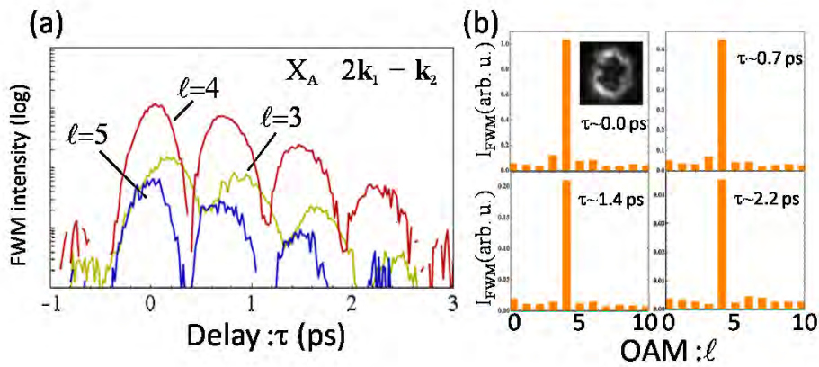
図 11: 励起光パルスに LG 光 ( \ell_1 = -2 , \ell_2 = 1 ) とした場合の (a) OAM 分解 FWM 信号光の時間発展と (b) コヒーレント振動ピークにおける OAM スペクトル。 \ell_{\text{FWM}} = 4 が支配モードである。
