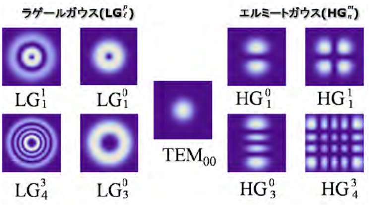
図 2: HG および LG モードの強度分布
