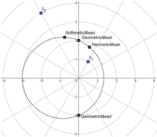
図 1: 4つの平均が調和点列であること。
