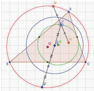
図 5: 外接円と九点円の 2 つの相似の中心
