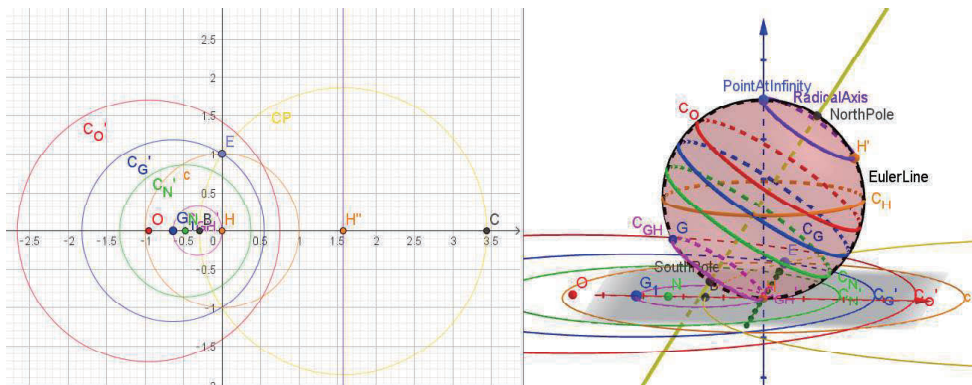
図 10: 立体射影で球面に引き戻した像
