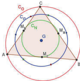
図 4: 外接円の重心円に関する鏡映は九点円である。
