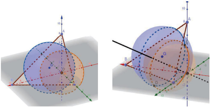
図 8: 3次元直交軸を利用した垂心円と重心円の作図
