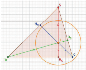
図 6: 方べきを考慮に入れた垂心円
