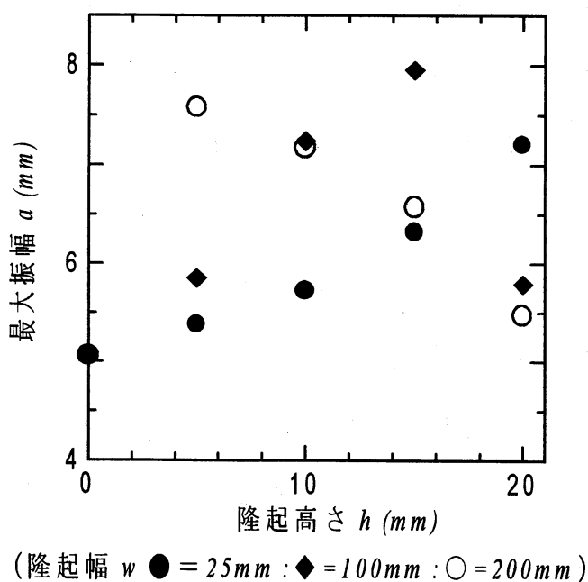
図 3 隆起高と最大振幅の関係
