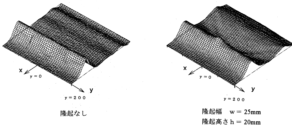
図4 隆起幅が小さいときの波形
