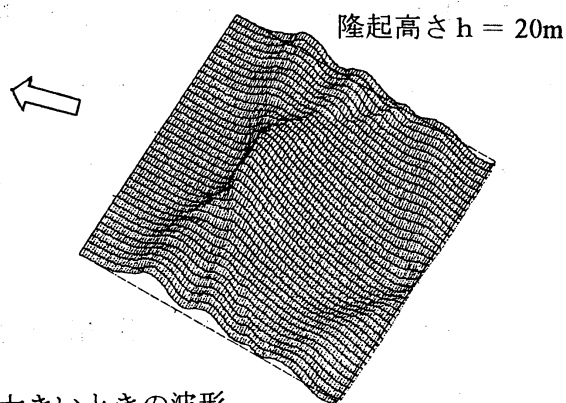
図6 隆起幅が大きいときの波形
