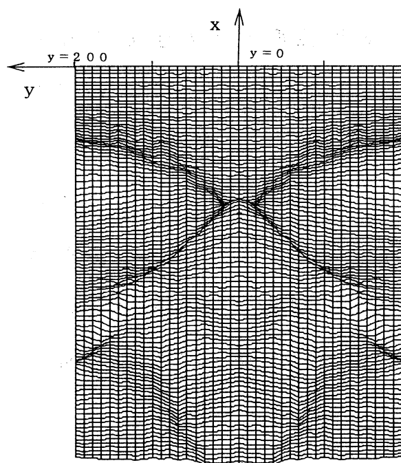
視点を変えた図 h = 20\text{ mm}
