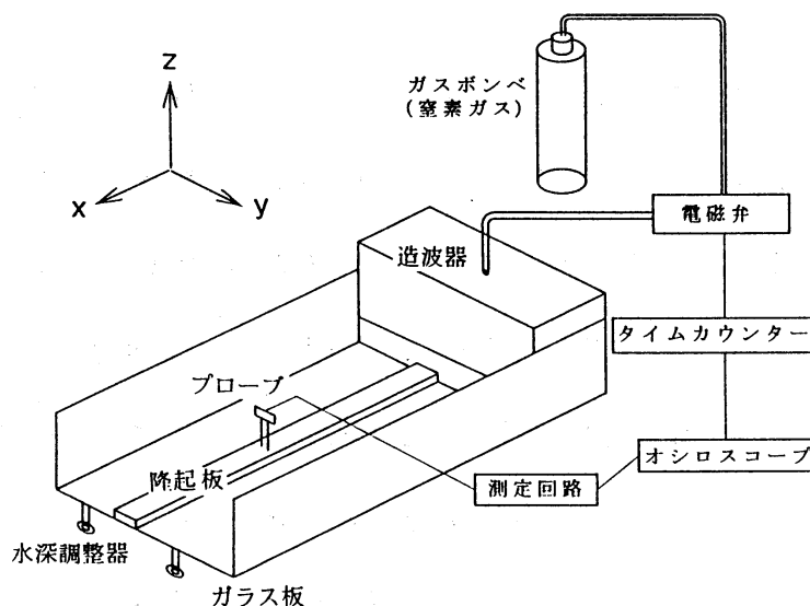
図2 実験装置図
