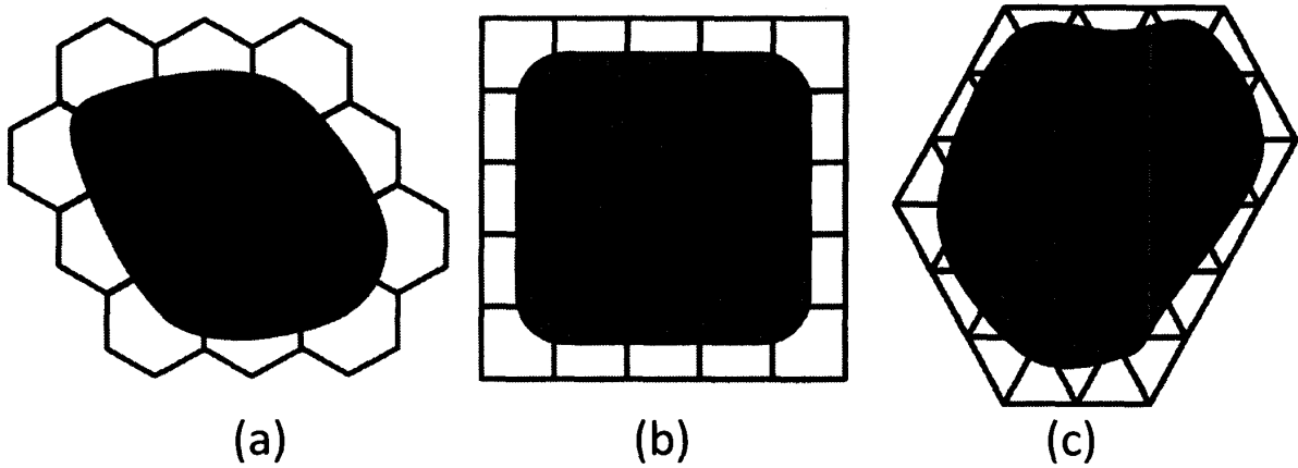
図 14: TPS の構造と面積則との対応, (a) 蜂の巣格子, (b) 正方格子, (c) 三角格子: いずれの結晶構造の場合も 16 サイトを含む部分系を切り出していますが, エンタングルメントが切れるボンド数には大きな違いがあります.
