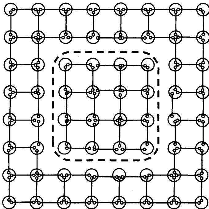
図 12: TPS の構造と面積則との対応: 非臨界系の面積則に合うようにエンタングルメント・ボンドが配置されている. 即ち, 点線で囲まれた領域 ( L=4, L^2=16 ) に対して, 部分系を区切ったことによって切れたエンタングルメント・ボンドの本数 N_{bond} = 4L = 16 が領域の長さを与えます. またそれによるエントロピー変化は N_{bond} \log \chi となります.
