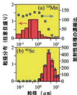
図2: 放射性核種の粒径とエアロゾル粒子への濃縮(溶融した放射性物質から生成した放射性エアロゾル粒子の例)
