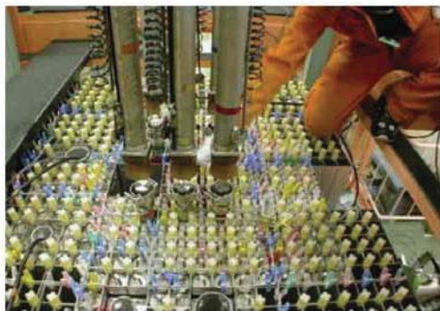
写真1: KUCAの固体減速炉心
