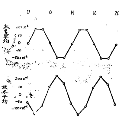
第7圖 阿蘇に於ける春夏、秋冬の平均半日變化(NS)
