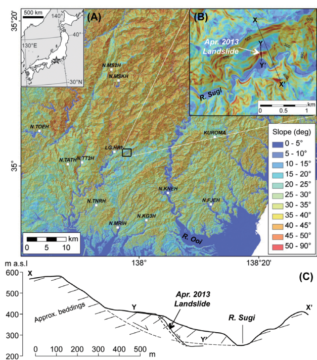
図 1 崩壊位置と周辺の地形および地形断面図 多数の地すべり地形が分布し、 30^\circ 以下の緩傾斜面が帯状に分布する泥質岩の卓越する地域の中に位置しており (A)、過去に南向きの受け盤斜面で発生した大規模崩壊の堆積物が蛇行河川によって攻撃された部分にあたる (B, C)。図 (A) 中には今回の崩壊起源の地震波が捉えられた地震観測点も示す。
