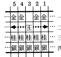
図 14: 左あるいは右へ追う部品
