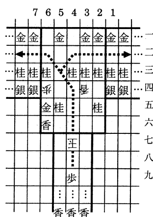
図 19: 入次数1 出次数2 の頂点に対応する部品 (後手選択)
