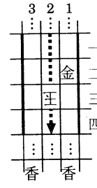
図 13: 下へ追う部品
