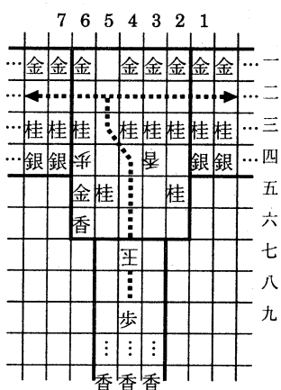
図 20: 入次数1 出次数2 の頂点に対応する部品 (先手選択)
