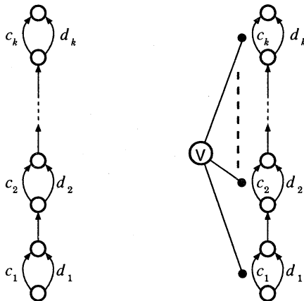
図 6: OR ユニット設置前 図 7: OR ユニット略記
