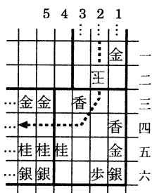
図 18: 下向きから左向きへ曲がって追う部品
