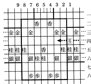
図 22: 入次数 2 出次数 1 の頂点に対応する部品 (二度目の進入時)
