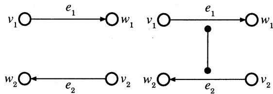
図 2: XOR ライン設置前 図 3: XOR ライン略記
