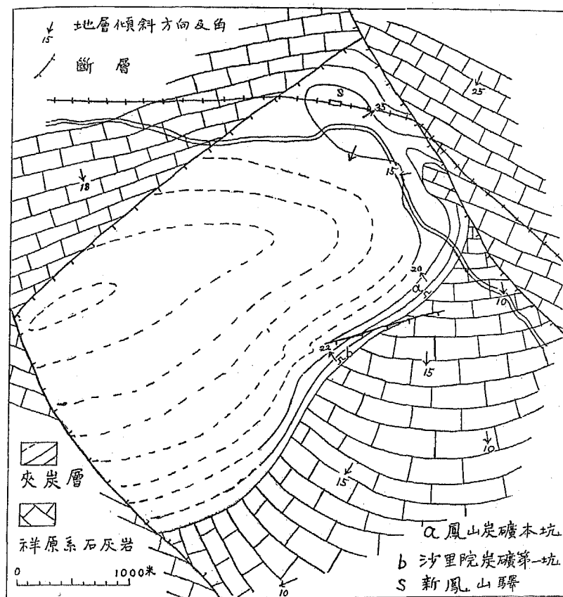
第一圖 鳳山炭田附近地質構造圖
