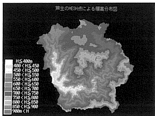
図4 高度別面積分布 Distribution of area in altitude
