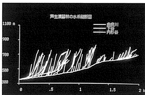
図7 水系縦断面図 Profile of streams
