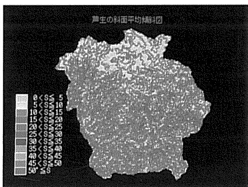
図6 メッシュ平均勾配図 Mean slope angle (50m x 50m mesh)
