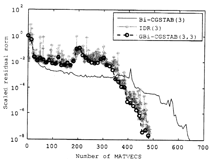
図7 s = L = 3 と設定した3つの手法の比較 (数値例2)
