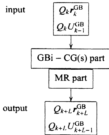
図 2 GBi-CGSTAB(s, L) の 1 反復
