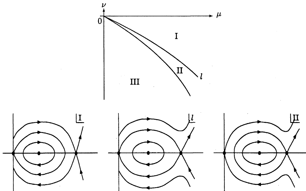
図 4: K = 0 超曲面上のダイナミクス
