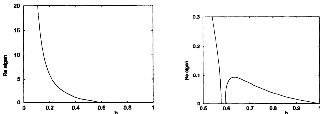
図 1: 左: 0 < b < 1 での E(b) のグラフ, 右: 左図の拡大
