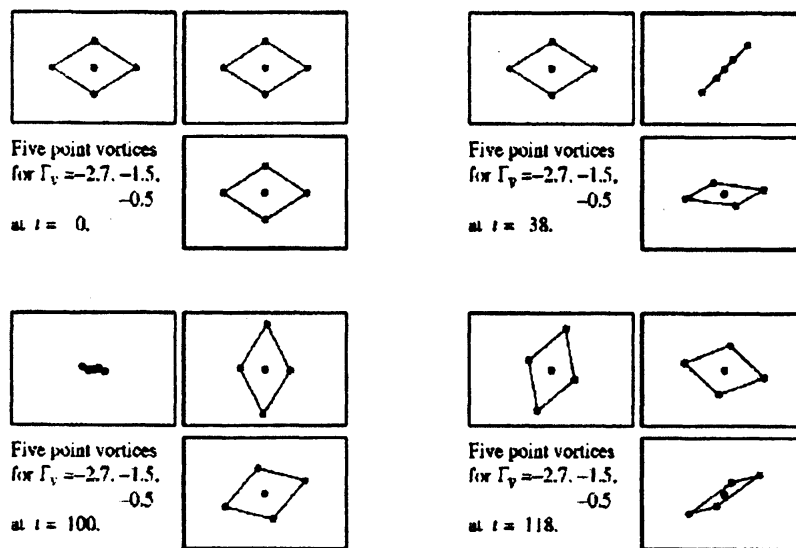
図 4: b = 0.6 , \Gamma_v = -2.7, -1.5, -0.5 での菱形形状の緩和振動の数値実験結果. 急激な動き (rapid motion) の際, 渦点が集まる範囲の違いが観測される. 特に, \Gamma_v = -2.7 のときは狭い範囲に集まっていることが分かる.
