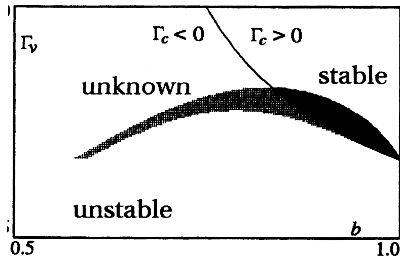
図 3: 相対的定常解が安定であることが検証可能なパラメータ領域（黒色の部分）と線形化不安定であるパラメータ領域（白色の部分）．灰色は elliptic であり，検証が失敗した領域を示す．
