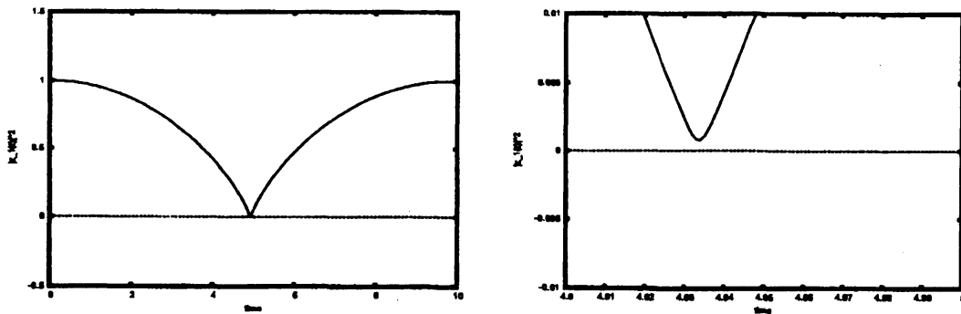
図 5: b = 0.6 , \Gamma_v = -1 のときの (12) の解 r(t) の時間変化. 左図を拡大したものが右図である.
