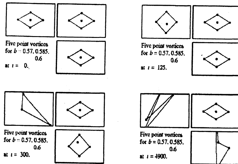
図 2: \Gamma_v = 1 での菱形形状下での数値実験結果 (動画を静止画にコマを落とした). b = 0.57, 0.585, 0.6 とした. b = 0.57, 0.6 の場合は不安定で形状が崩れるが, b = 0.585 の場合は長時間, 初期形状を保つことが分かる.
