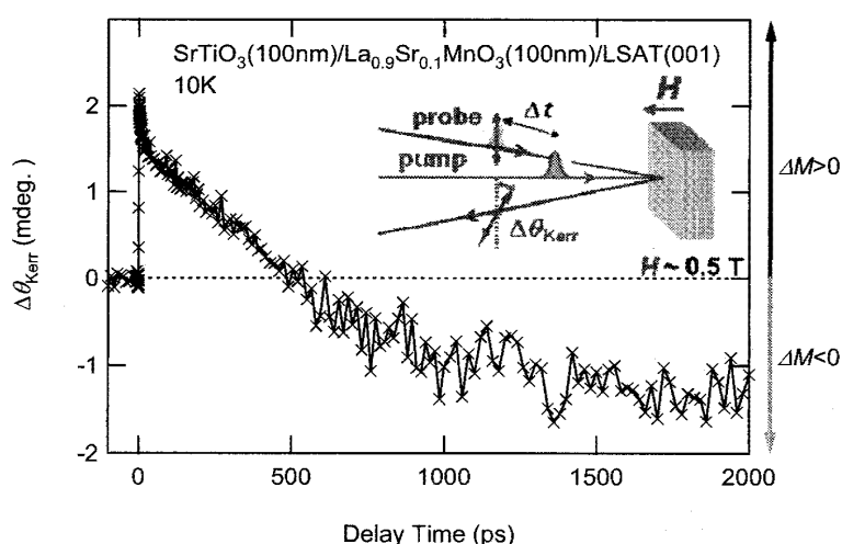
図 \text{SrTiO}_3/\text{La}_{0.9}\text{Sr}_{0.1}\text{MnO}_3/\text{LSAT} における \Delta\theta_{\text{Kerr}} の時間変化(10K)と実験配置
