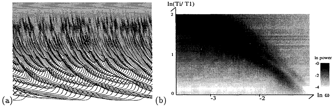
図 3: モデル式 (3) で、 T_{total} = 100, L = 100 として、最上流に微小ノイズを加えた場合の時空プロット (a) を示す。(b) はそれらの素子のパワースペクトルをグレースケール表示で示す。色が濃い程、値が大きい。
