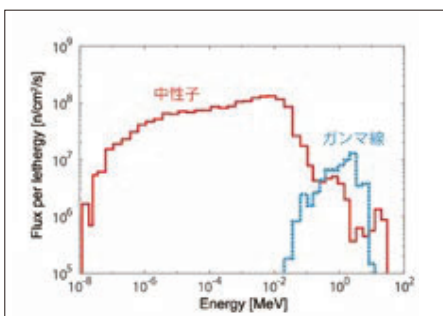
BNCT照射場の中性子和ガンマ線スペクトル
