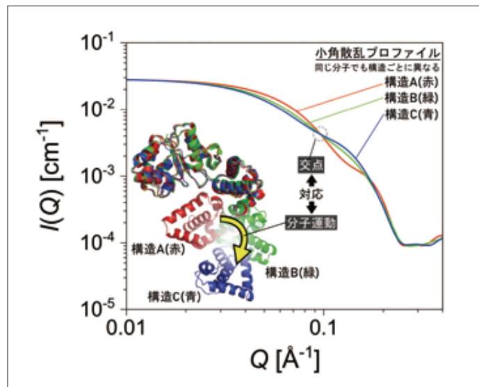
小角散乱プロファイルを用いた生体分子運動解析
