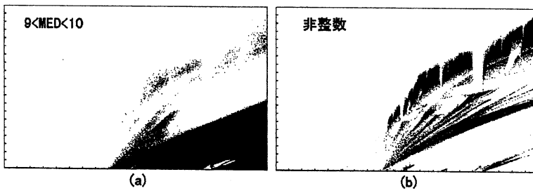
図 7 (a) 9 < MED \leq 10 となる領域. (b) 1 < MED < 9 で非整数のものの領域. 横軸は 1.0 \leq a \leq 2.0 , 縦軸は 0.0 \leq \varepsilon \leq 0.5 .
