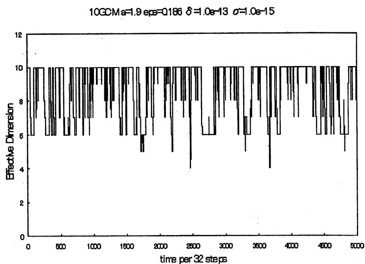
図 10 10GCM の有効次元の変化. a=1.9 , \epsilon=0.186 , 有効次元の精度 \delta=10^{-13} 、ノイズの大きさ \sigma=10^{-15} 、倍精度で計算。ランダムに与えた初期値 x(0) \in R^{10} の軌道を x(t) とし、点 x(t) における有効次元 ED(x(t), \delta) を 32 ステップ毎に 5000 回記録したもの。
