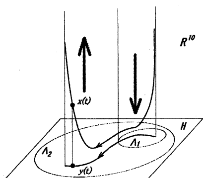
図 20 カオス遍歴のメカニズムの概念図。射影点 y が「擬アトラクタ」 \Lambda_1 の内部を動くとき、直交補空間方向に安定であるから、 x は H に接近する。射影点 y が「擬アトラクタ」 \Lambda_1 の出口を見つけ、外に出て \Lambda_2 の内部を動き回ると、直交補空間方向は不安定となり、 x は H から離れる。
