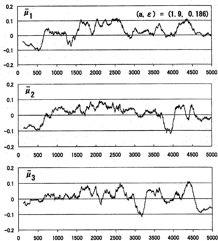
図 14 重み[322111]付き 6 GCM における局所横断 Lyapunov 数の変化。 a=1.9, \epsilon=0.186 , ノイズの大きさ \sigma=10^{-15} 。
