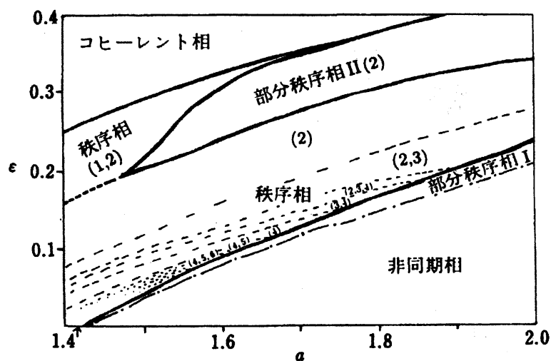
図2 金子氏による GCM の相図. N=200. (金子邦彦・津田一郎 著, 「複雑系のカオス的シナリオ」 複雑系双書 1, 朝倉書店, 1996. P.134 からの転載)
