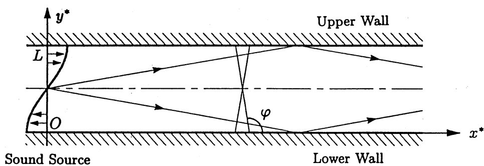
図 5. 二次元導波路を伝播する第一モードの音波 (概念図). 矢印は線形波の波数ベクトルの方向 [(19) 参照]. \varphi = \pi - \arctan(\Omega\kappa/\pi) は線形波の波面と x 軸のなす角度.
