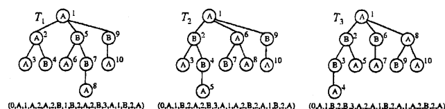
図 3: ラベルつき順序木の深さラベル列
