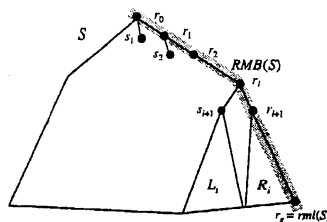
図 4: 正規形表現に関する記法
